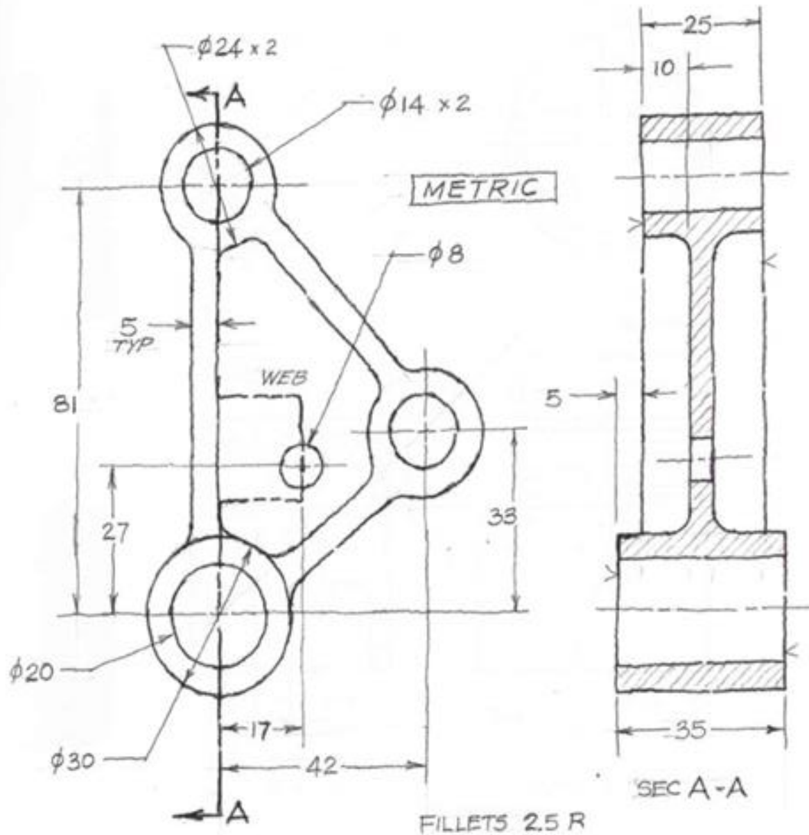
Shift link
